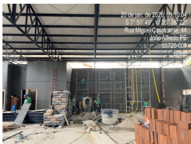
FOTO 11: Montagem, escoramento e concretagem das paredes de PVC.
